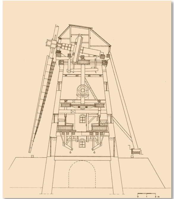
Doorsnede stenen bergmolen. Bron: Korenmolens, van Ambacht tot Industrie . Bewerkt door: @Rob
